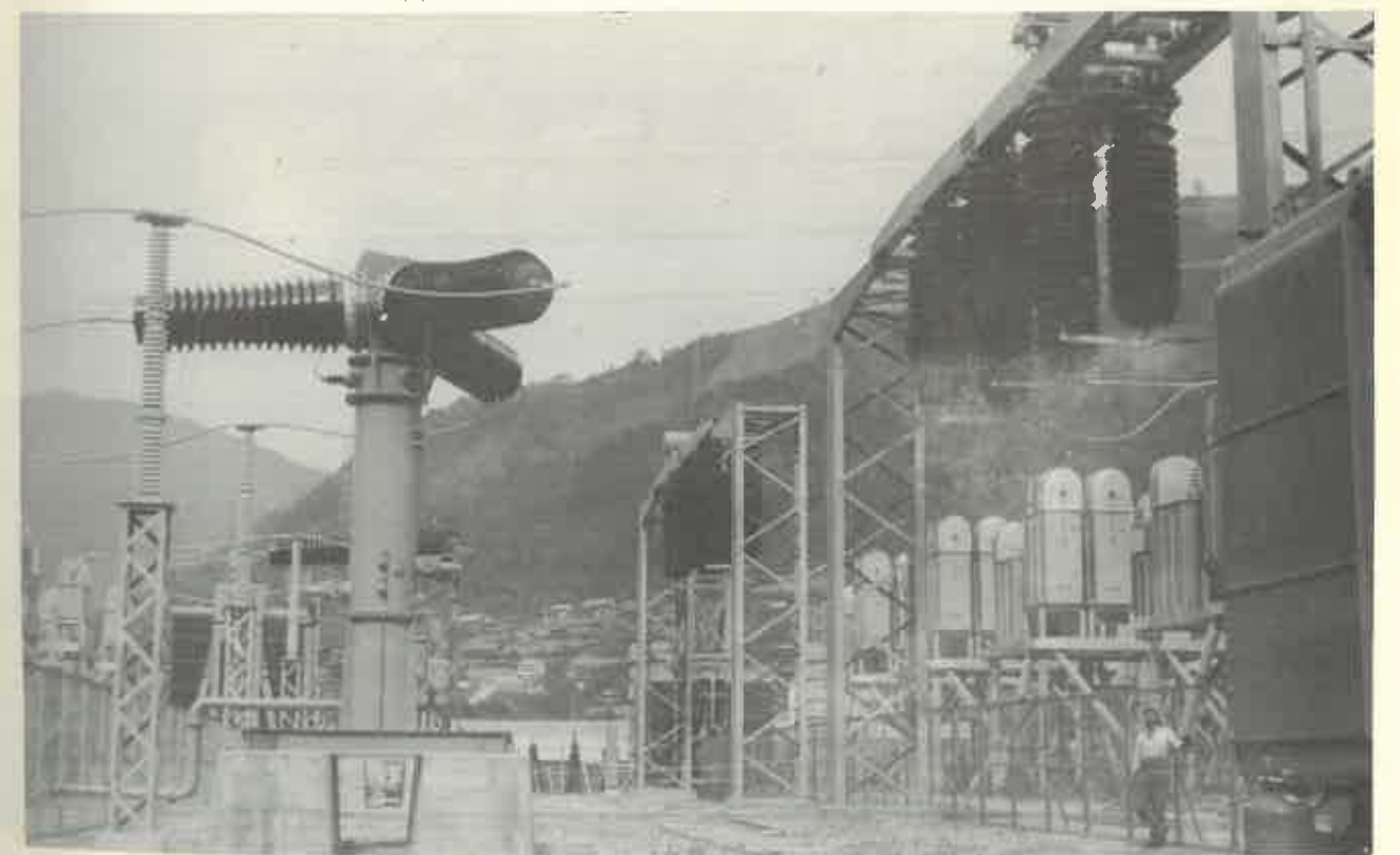
▲50%第13, 高次高周波フィルタリアクトル抵抗器
