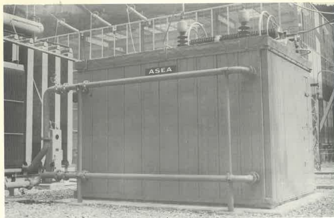
▲直流リアクトル上屋
