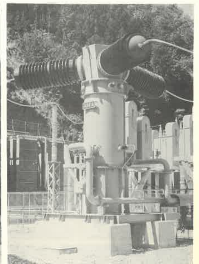
▲50%第7高調波フィルタリアクトル抵抗器
