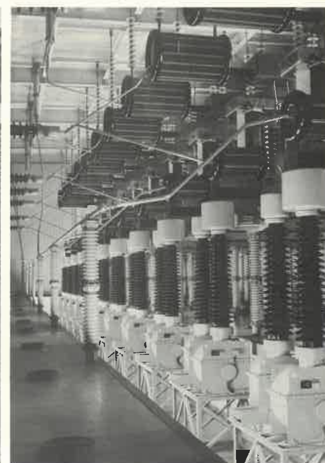
▲絶縁変圧器, 陽極リアクトル, 陰極リアクトル
