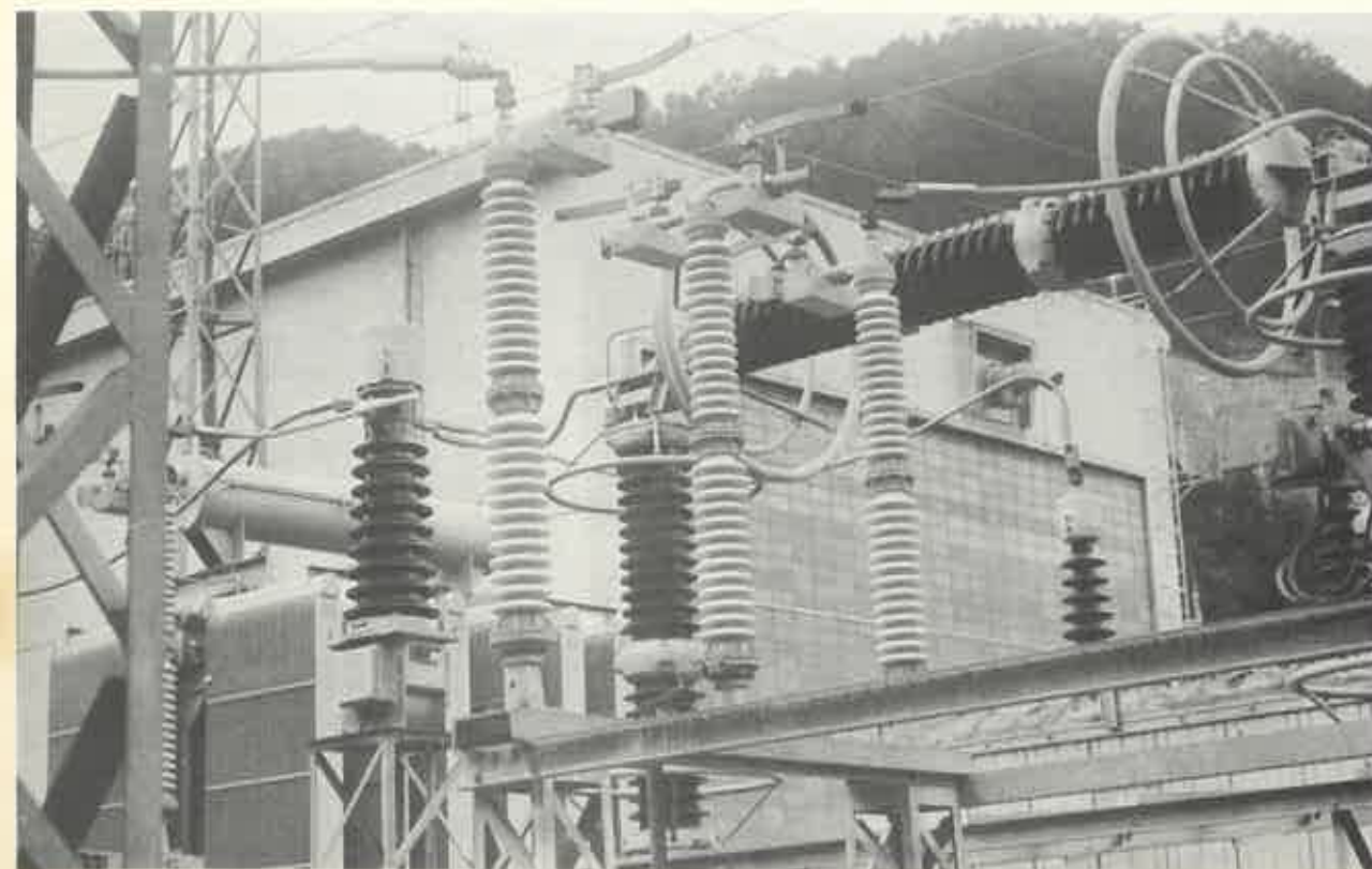
▲バイパス断路器
