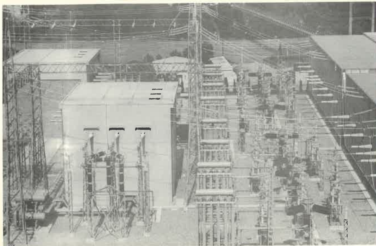
▲50%, 60% 主要変圧器上屋, バルブGR. 4用相間, 対地避雷器および振動防止防止回路
