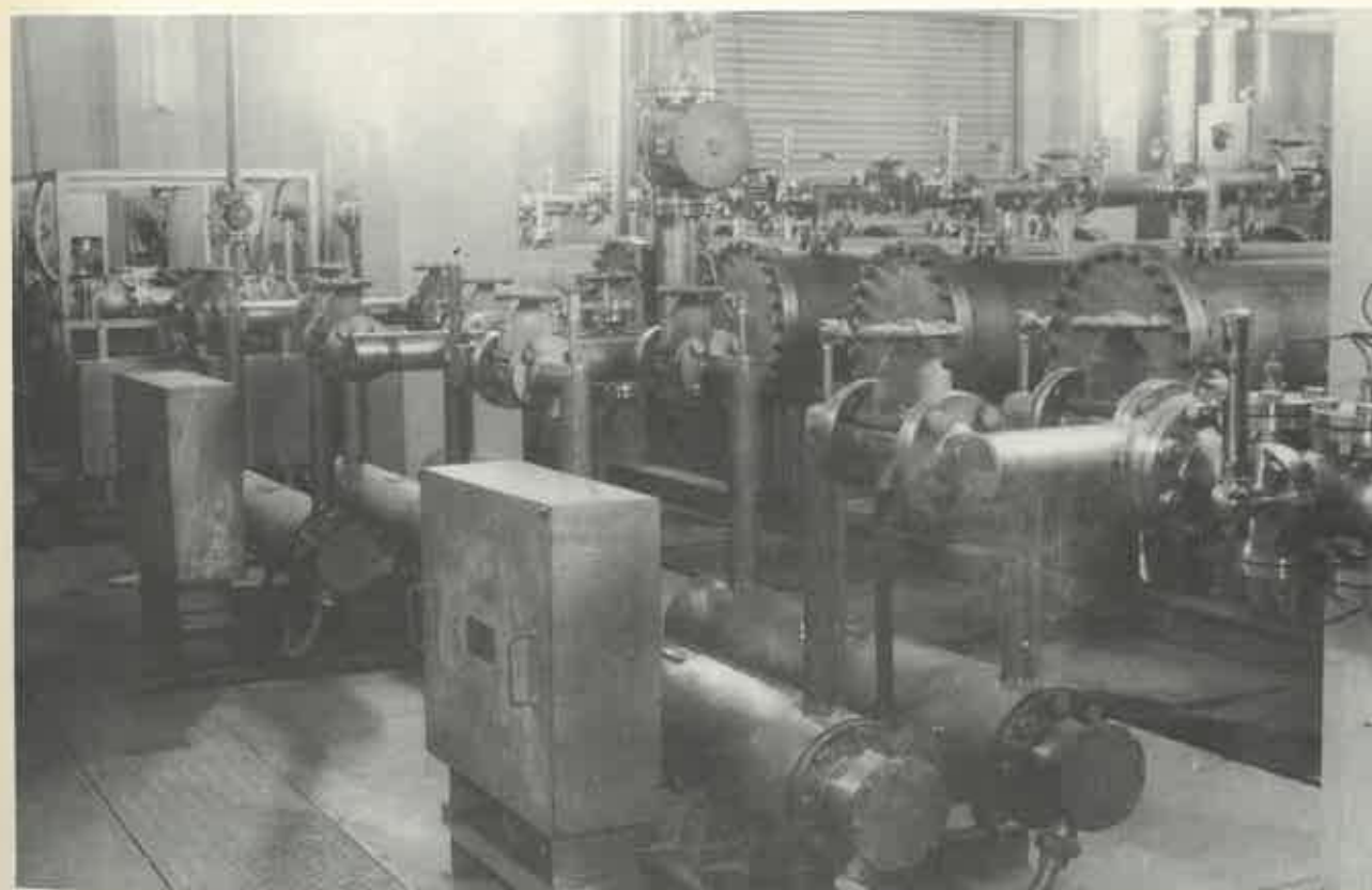
▲純水冷却設備
