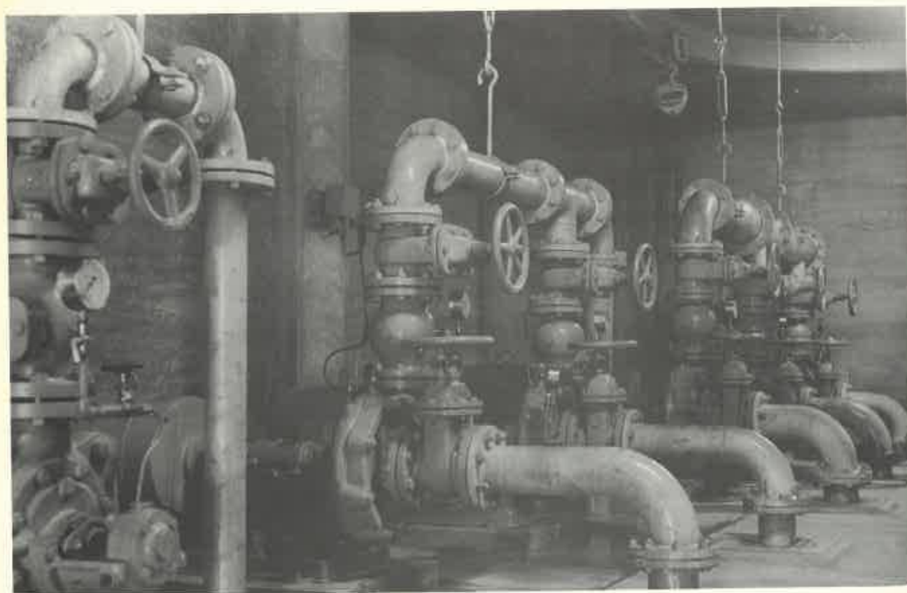
▲純水冷却設備給水用ポンプおよび空調設備給水用ポンプ
