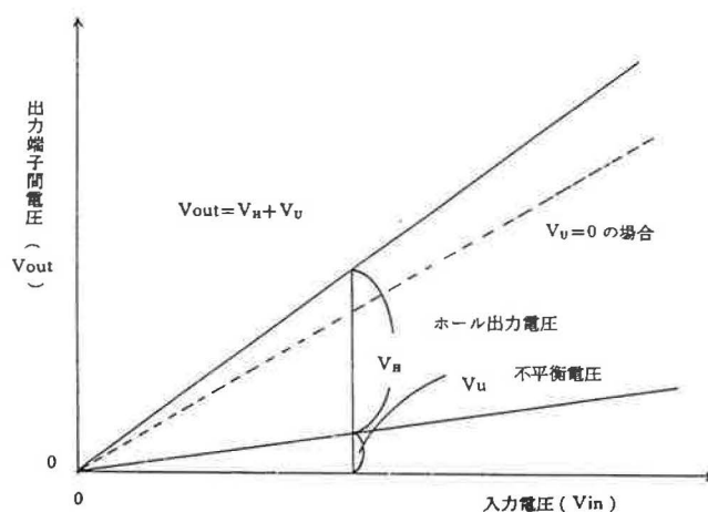
図3 ホール素子の入力電圧と不平衡電圧、ホール出力電圧の関係（磁束密度＝一定）
