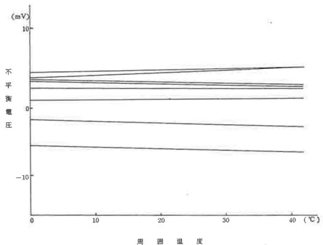
図21 不平衡電圧の温度変化 (1 V 定電圧)
