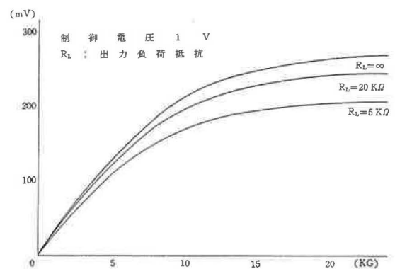
図15 ホール素子 出力電圧—磁界特性
