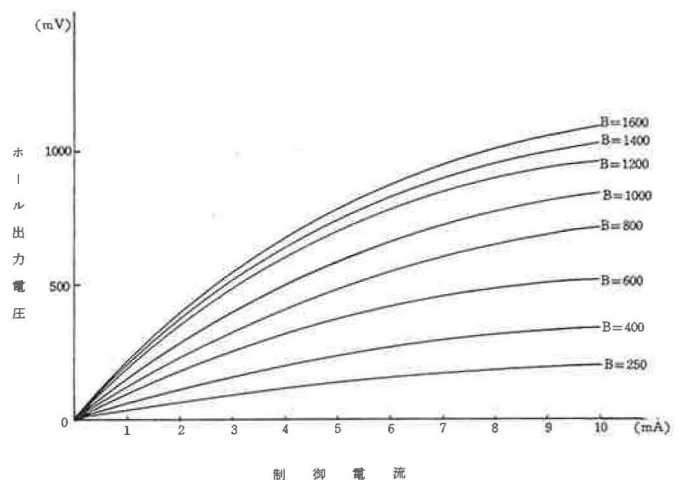
図22 ホール素子 出力電圧－制御電流特性
