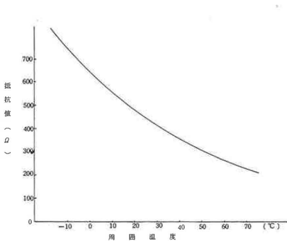
図20 ホール素子の入力抵抗の温度変化
