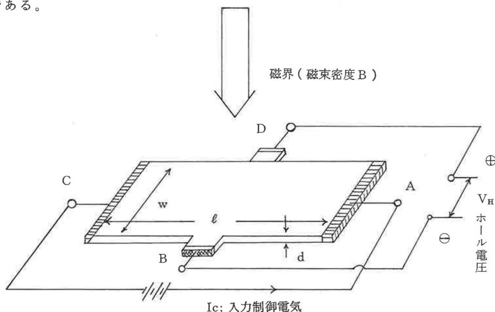
図1 ホール素子のホール効果
